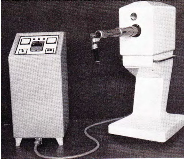
FIGURA 4. Segon fotocoagulador Olivella-Garrigosa, que emprava una bombeta de gas xenó (1965). A l'esquerra, l'equip elèctric i, a la dreta, l'equip òptic 5
