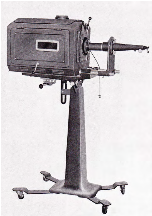
FIGURA 2. Primer fotocoagulador Olivella-Garrigosa, d'arc de carbons (1955) 5
