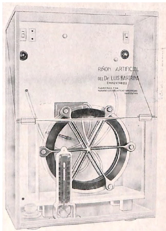
FIGURA 7. Darrera versió (any 1958) del ronyó artificial de Bartrina 3
