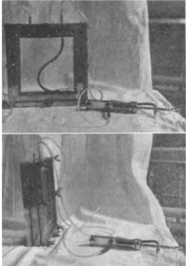
FIGURA 3. Cèl·lula dialitzant del primer aparell de Bartrina, en visió frontal (superior) i lateral (inferior) 15
