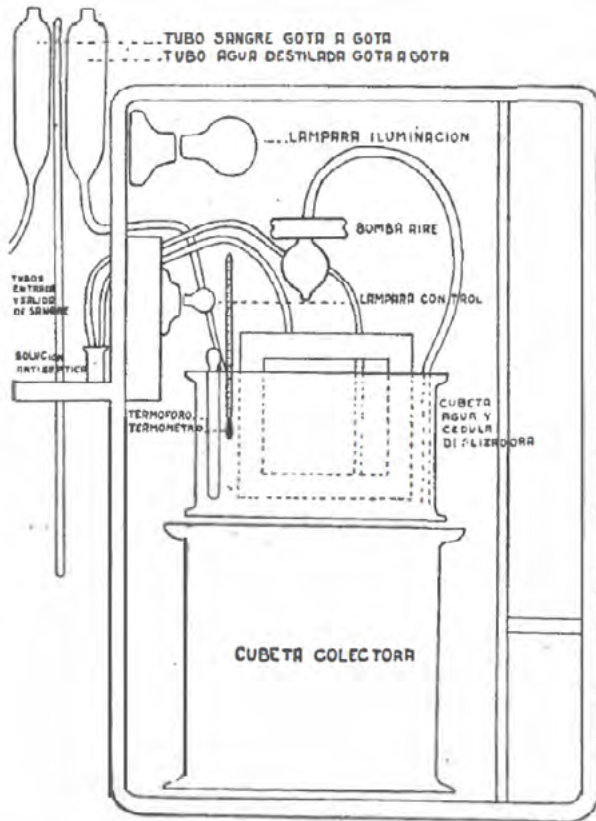
FIGURA 4. Esquema de l'aparell que Bartrina emprà inicialment com a ronyó artificial 15
